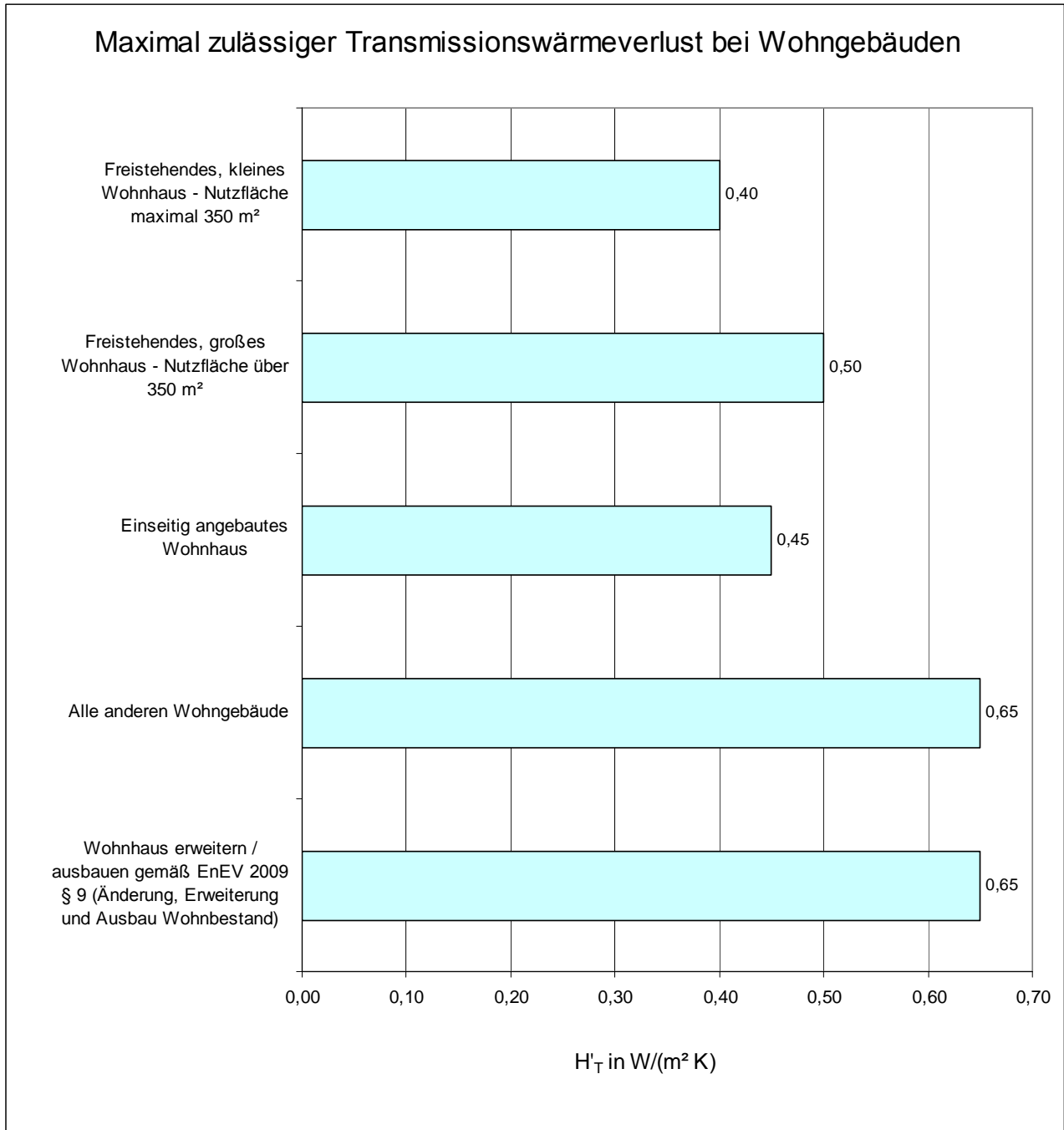
Grafik 1: Anforderungen der EnEV 2009 an den Wärmeschutz der Gebäudehülle bei neuen Wohngebäuden. Höchstwerte des spezifischen, auf die wärmeübertragende Umfassungsfläche bezogenen Transmissionswärmeverlusts.
